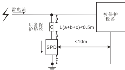
一般接线
